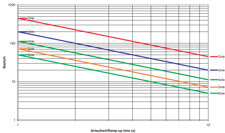
VersiStart II 400-25
